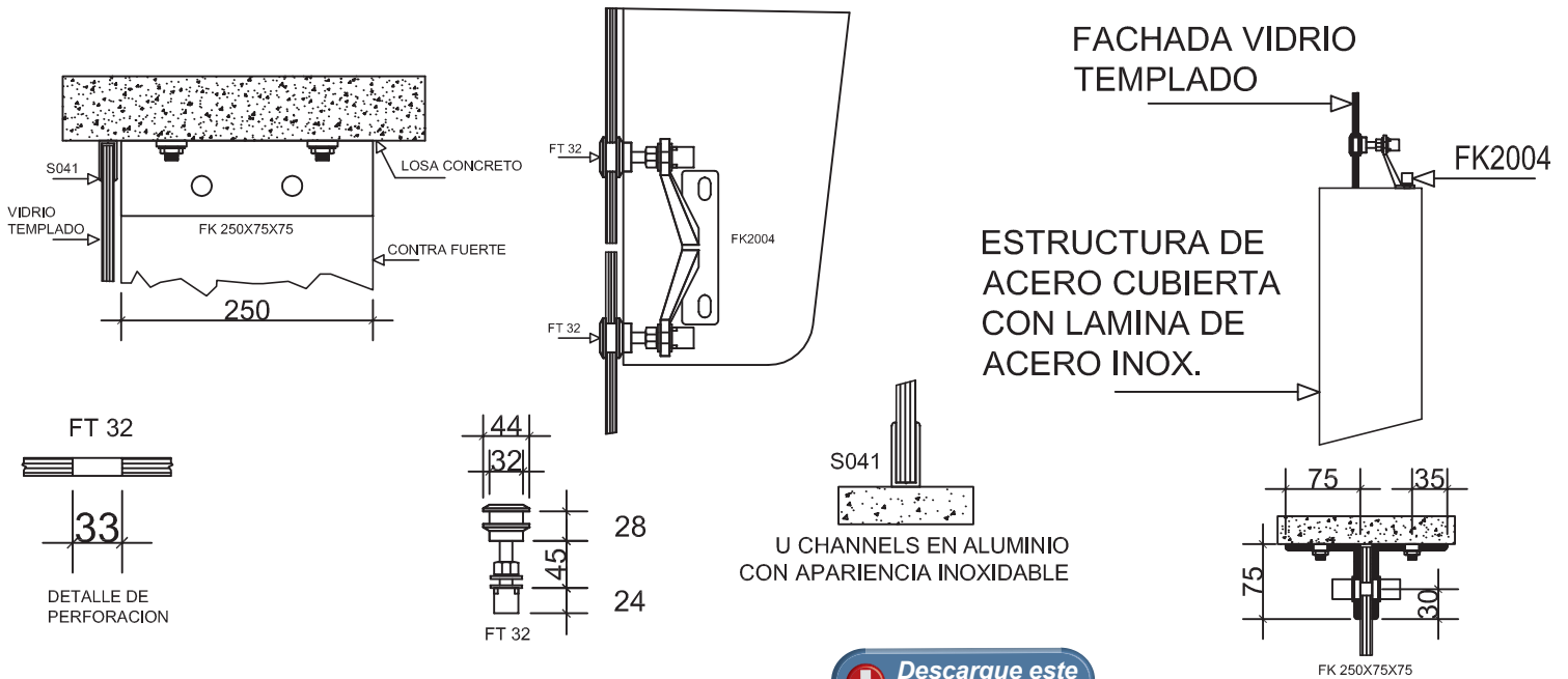
ELEVACION FRONTAL
